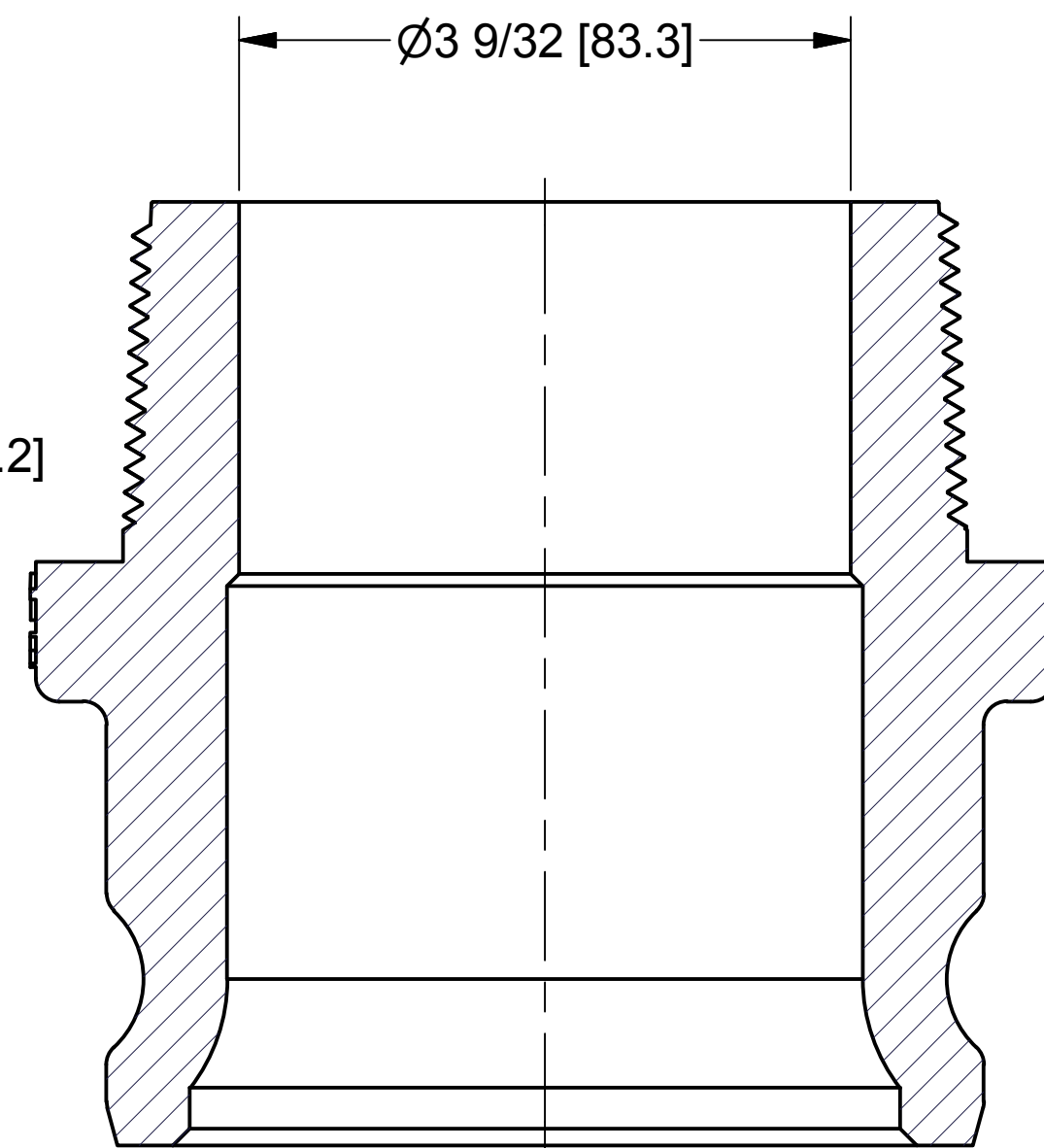
SECTION D-D SCALE 1 : 1
