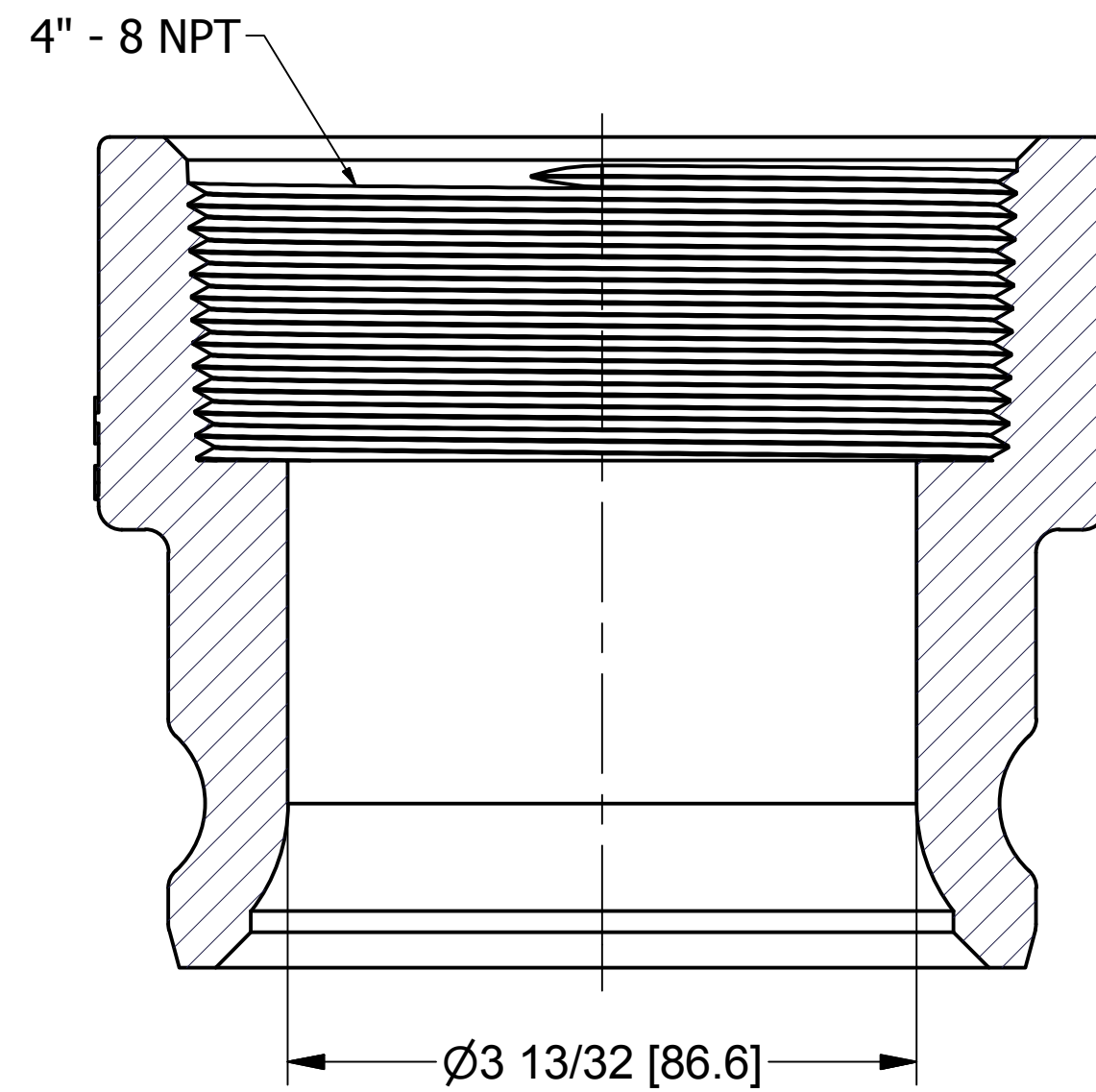
SECTION D-D SCALE 1 : 1
